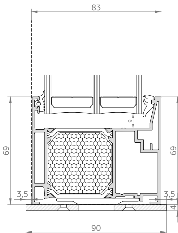
6993CC ALU PODLOGA PRAGA ZA STAROGRANJE 90 mm - NERO
