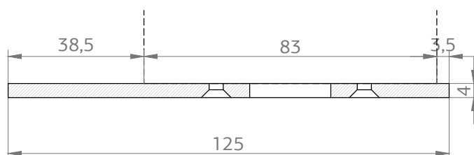
6995CC ALU PODLOGA PRAGA ZA STAROGRANJE 125 mm - NERO
