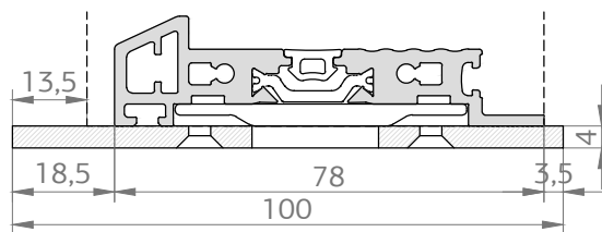
6994CC ALU PODLOGA PRAGA ZA STAROGRADNJE 100 mm - NERO
