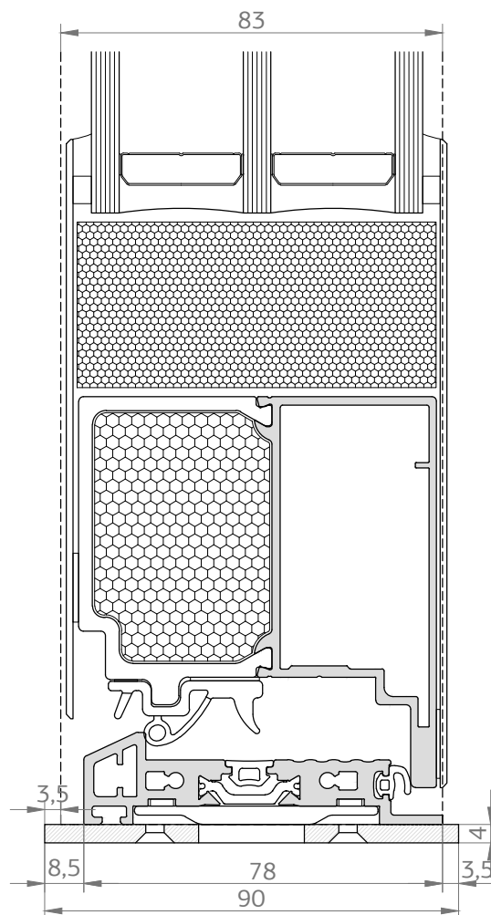
6993CC ALU PODLOGA PRAGA ZA STAROGRADNJE 90 mm - NERO
