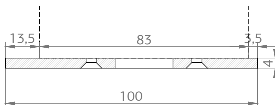
6994CC ALU PODLOGA PRAGA ZA STAROGRANJE 100 mm - NERO
