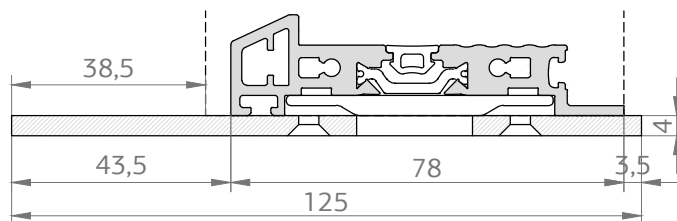
6995CC ALU PODLOGA PRAGA ZA STAROGRADNJE 125 mm - NERO
