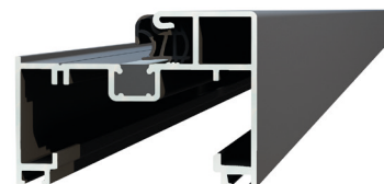
Thermo-ALU-Zarge mit thermischer Trennung (ATU56)
