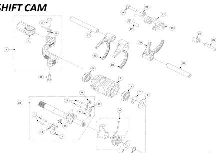
SELECTOR DE CAMBIO SHIFT CAM
