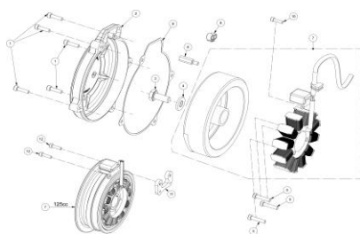
ENCENDIDO IGNITION
