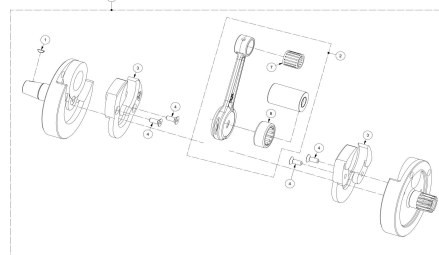
CIGUEÑAL CRANKSHAFT
