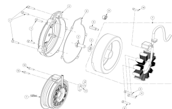
ENCENDIDO IGNITION
