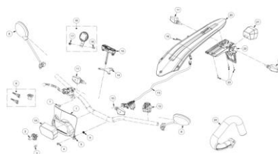
CHASIS FRAME
