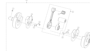
CIGUEÑAL CRANKSHAFT
