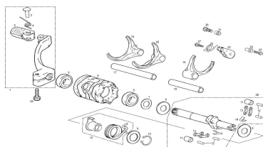
SELECTOR DE CAMBIO SHIFT CAM
