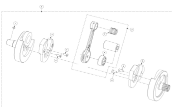
CIGUEÑAL CRANKSHAFT
