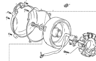
ENCENDIDO IGNITION
