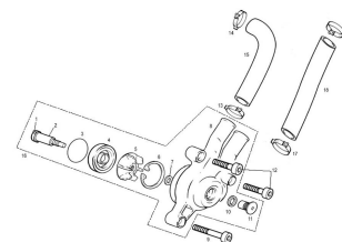
BOMBA DE AGUA WATER PUMP
