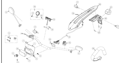
CHASIS FRAME
