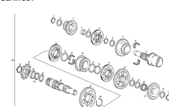
ENGRANAJES CAMBIO GEAR SET
