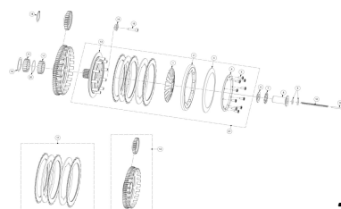
EMBRAGUE CLUTCH
