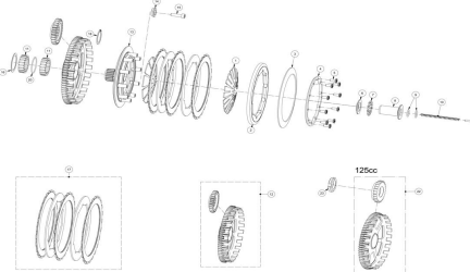
EMBRAGUE CLUTCH
