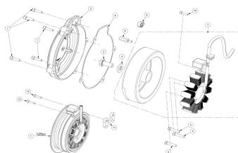
ENCENDIDO IGNITION
