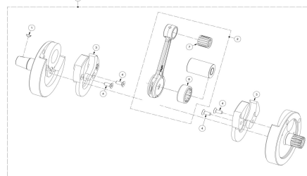
CIGUEÑAL CRANKSHAFT
