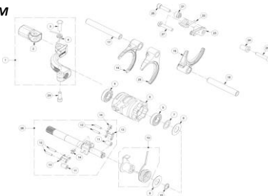
SELECTOR DE CAMBIO SHIFT CAM
