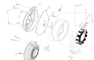
ENCENDIDO IGNITION
