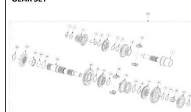
ENGRANAJES CAMBIO GEAR SET
