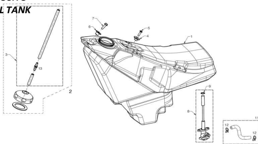
DEPÓSITO FUEL TANK
