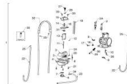
CARBURADOR CARBURATOR
