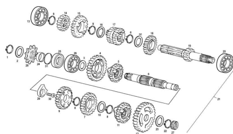
ENGRANAJES CAMBIO TRANSMISSION
