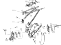
SubFrame
