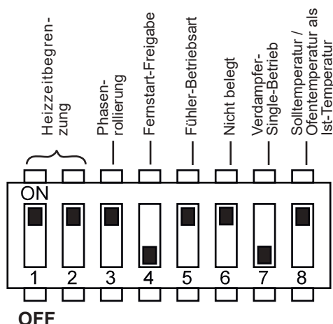
Abb.6 Funktionswahlschalter - Standardeinstellung
