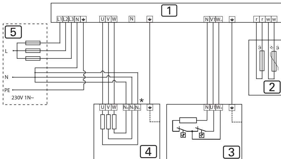
Kuva 6 Liitântäkaavio, malli 230 V 1N~ Home combi 6,0 kW ja 9,0 kW (HOME-C60 / HOME-C90)
