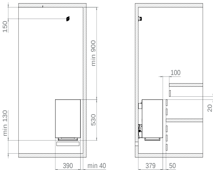
Bild 1 Säkerhetsavstånd Home combi 6,0 kW och 9,0 kW (HOME-C60/HOME-C90) Mått i mm
