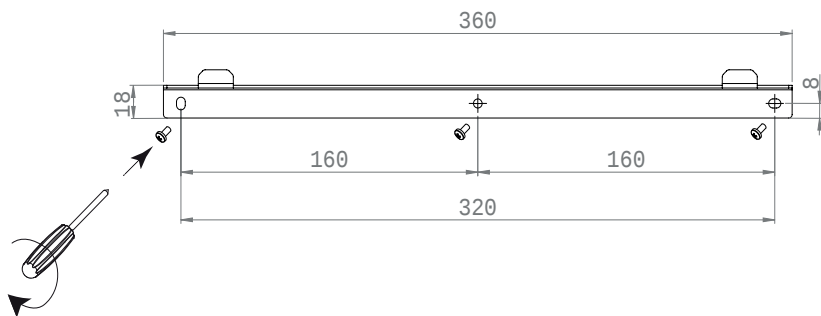
Abb.2 Montageleiste Home combi
