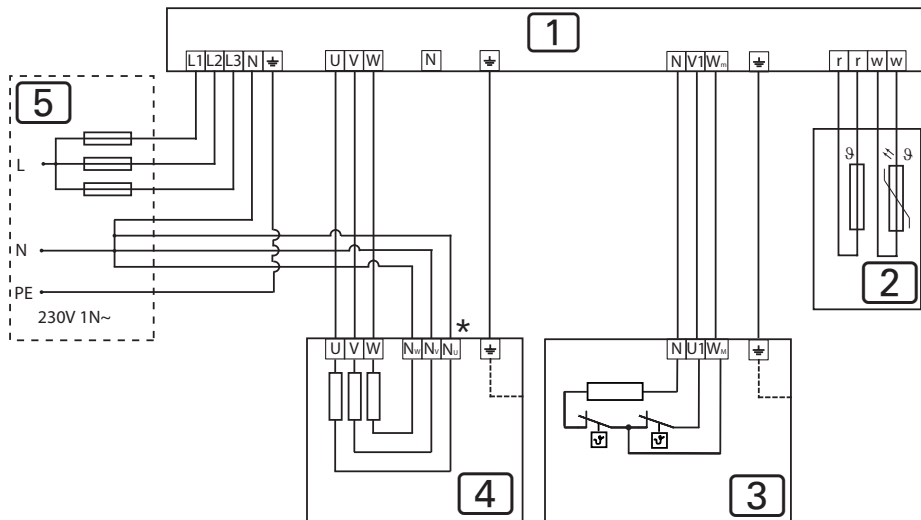
Bild 6 Kopplingsschema 230 V 1 N~ Home combi 6,0 kW och 9,0 kW (HOME-C60/HOME-C90)
