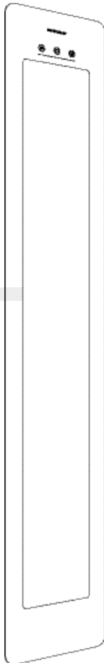
Sunshower ONE /L - IR Sunshower PLUS /L - IR+UV Glas - L 1850 x B 330 mm Eingebaute Maße - H 1769 x B 263 mm Unterputz / Aufputz gerade Wand + Ecke
