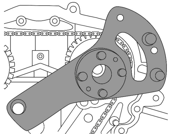
Árbol de levas de entrada
