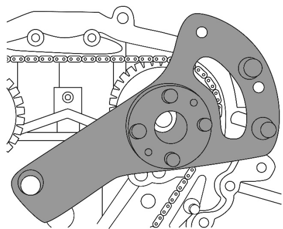
Einlass-Nockenwelle
