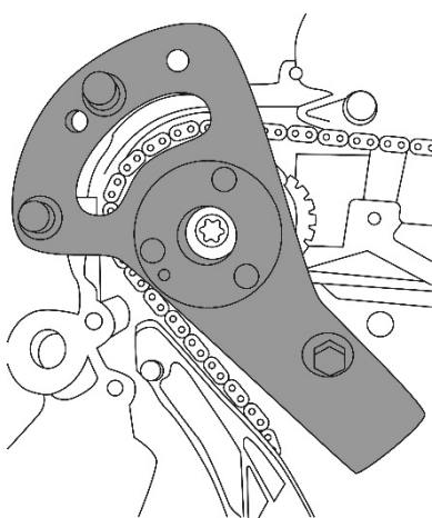
Auslass-Nockenwelle
