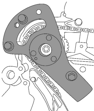
Árbol de levas de escape
