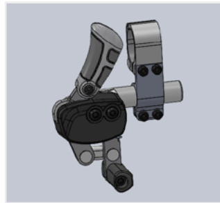
// QSF060002 Kniehebelbremse
