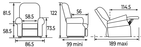
Abstand** von der Wand: 66 cm
