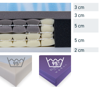
TreviraCS-Spannbezug
