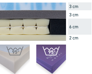
TreviraCS-Spannbezug
