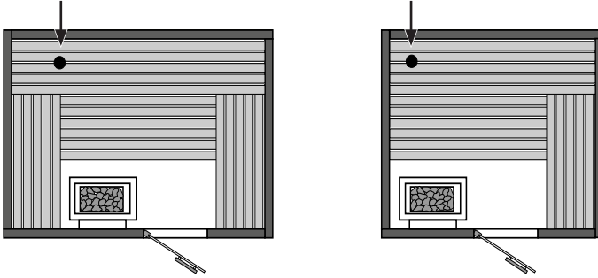
Einbauposition Bankfühler
