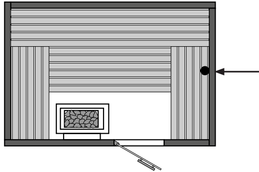
Montageposition Feuchtfühler
