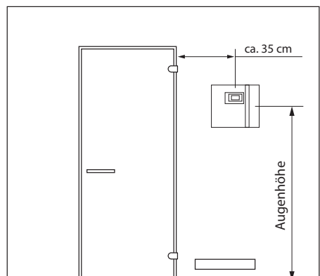
Montage an der Kabinenwand
