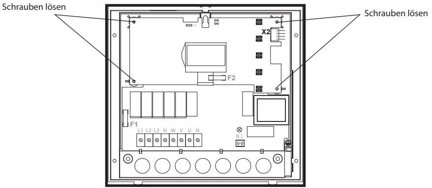
Display-Platine
