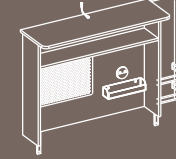
DAR ÇALIŞMA ÜNİTESİ NARROW STUDY UNIT G:108.5 x Y:72 x D:29 cm 20.58.1102.00
